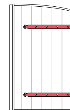
Sans barre ni écharpe avec contre-pentures blanches ou noires
