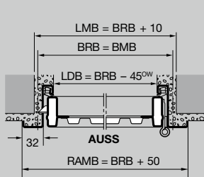
Coupe horizontale
