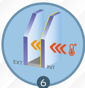
6 DOUBLE VITRAGE 28 mm 4/20/4 avec couche ITR, remplissage gaz argon et intercalaire WarmEdge faible émissivité
