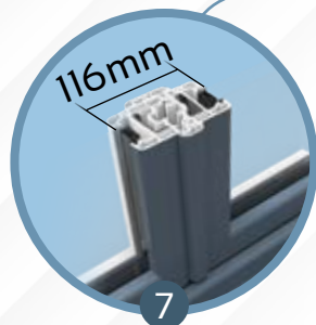
7 BATTEMENT EXTÉRIEUR réduit et habillé
